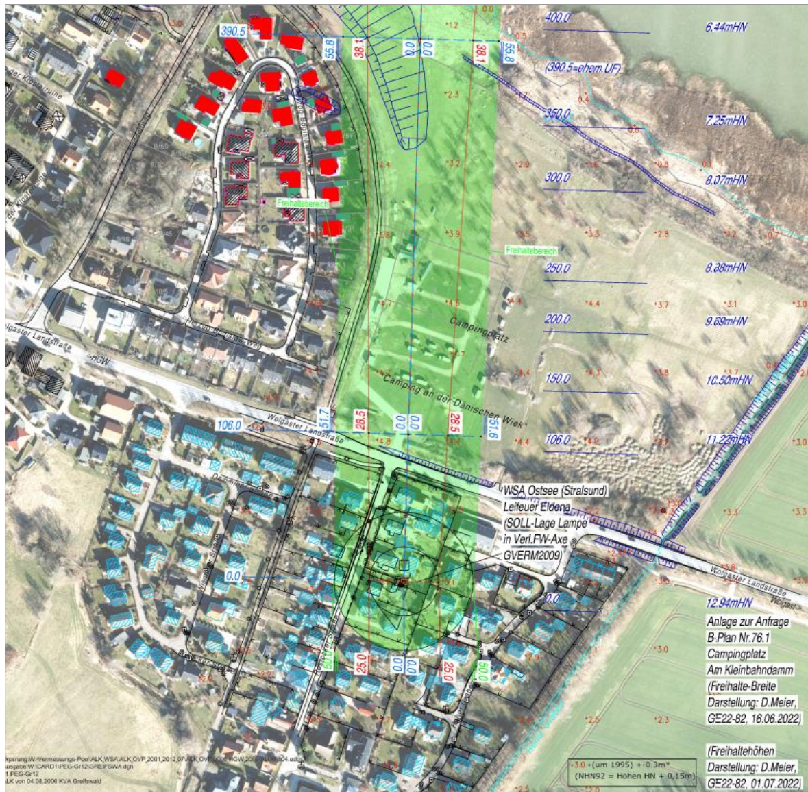
Abbildung 11: Freihaltezone des Leitfeuers Eldena
